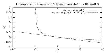
Figura 2: O significado relativo da linearização
