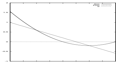
Figura 1: gráfico de f e de uma tangente.
